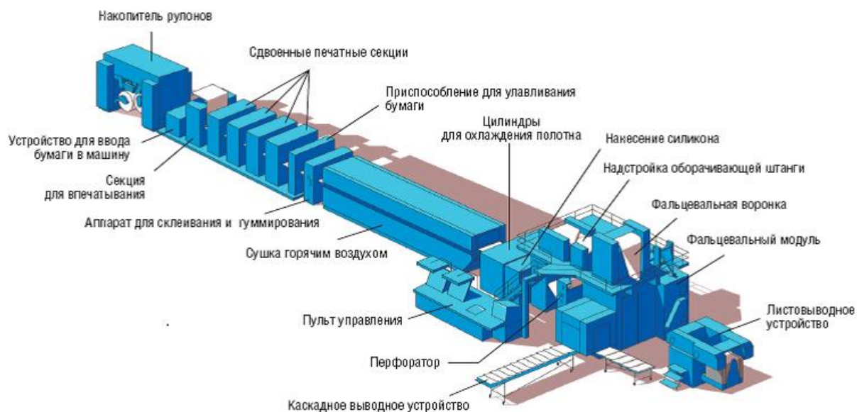
Рулонная печатная машина М-600 с опцией листовой выклад (на рисунке справа).
