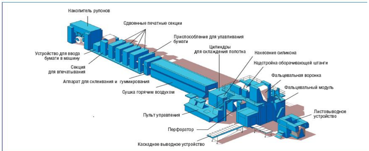
Рулонная печатная машина М-600 с опцией листовой выклад (на рисунке справа).
